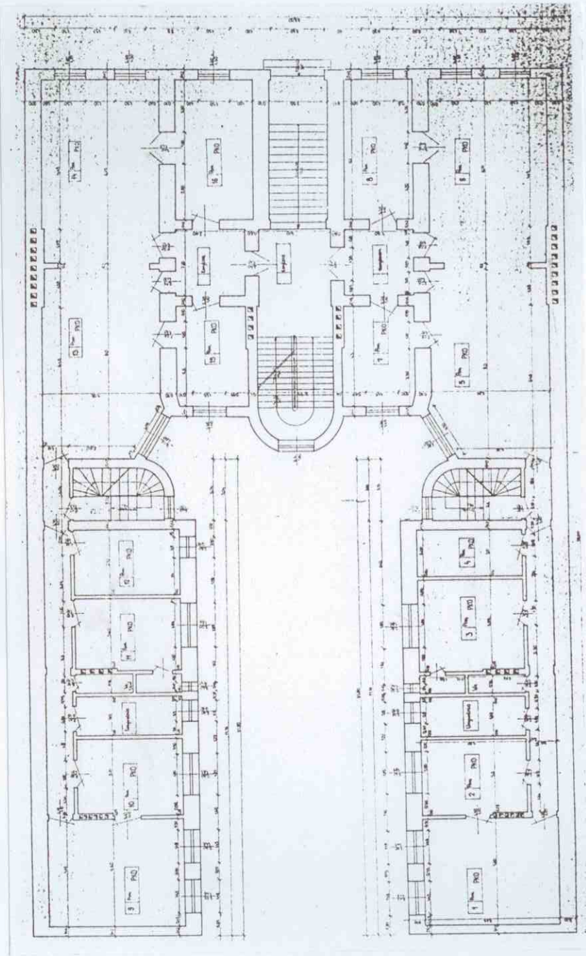
RZUT PARTERU
